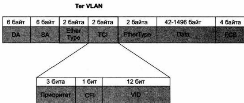
Рисунок 5 – Структура помеченного кадра Ethernet
