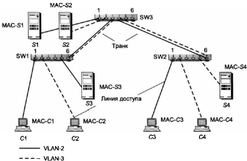
Рисунок 6 – Разбиение сети на две виртуальные локальные сети
